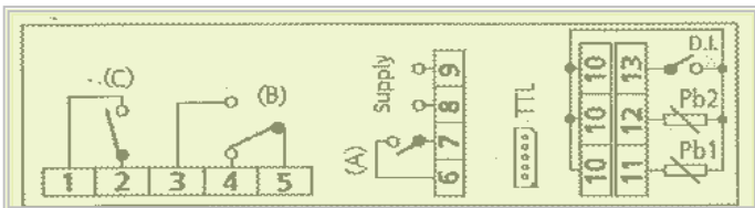
Shéma du Thermostat
